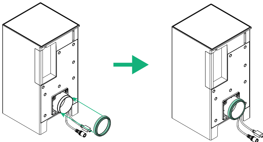
Anneau d'étanchéité
