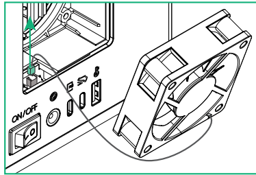
Lepaskan konektor
