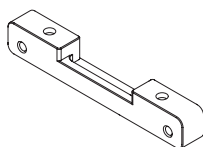
固定具B
