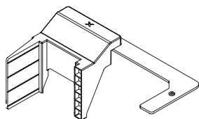
Peça limitadora
